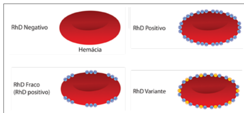
Figura 4 – Esquema do RhD, D fraco e D variante
